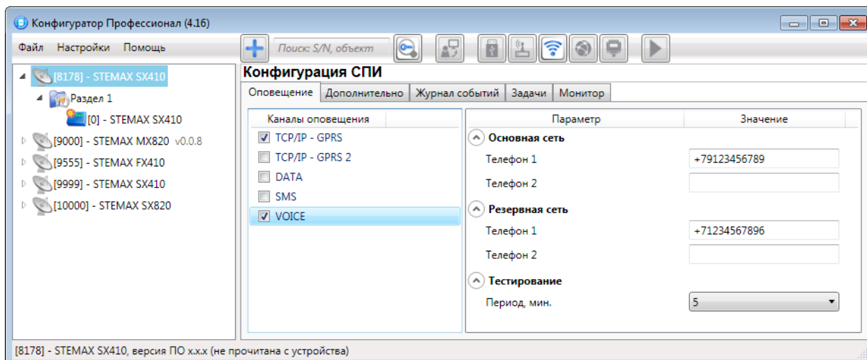
Рис. 5.10. Параметры канала VOICE
