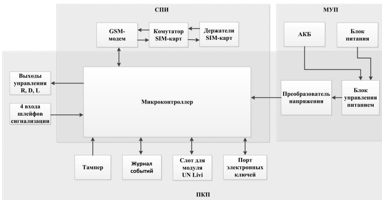
Рис. 3.1. Функциональная схема
