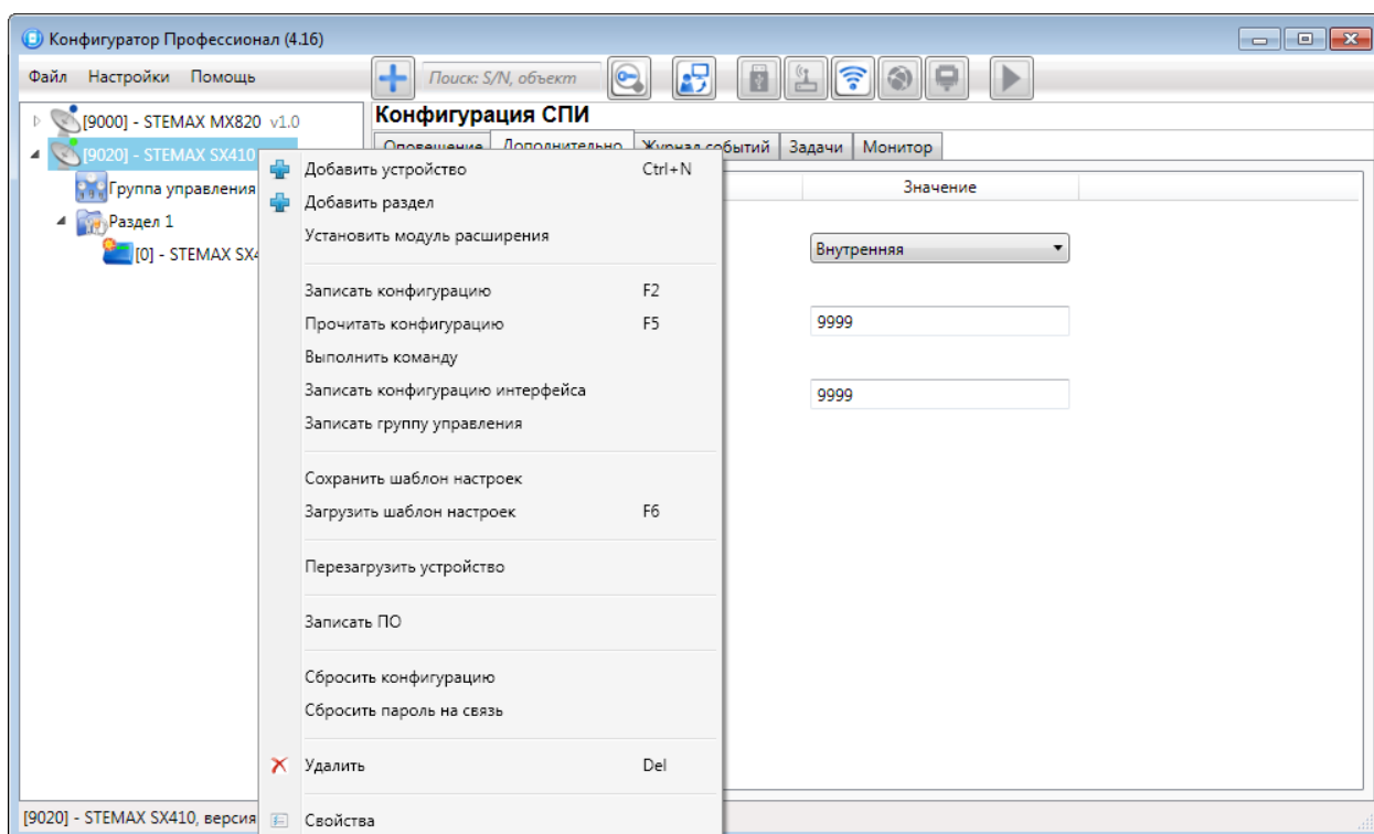
Рис. 6.1. Контекстное меню контроллера
