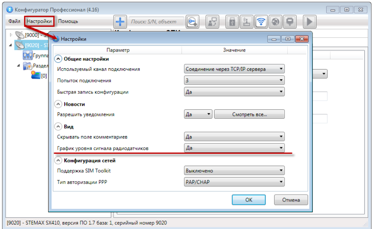
Рис. 5.17. Включение функции отображения графика уровня сигнала радиоустройств
