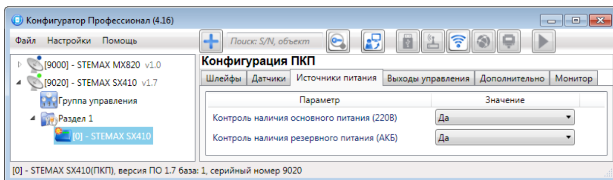
Рис. 5.31. Вкладка Источники питания
