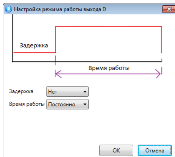
Рис. 5.34. Окно Настройка режима работы выхода
