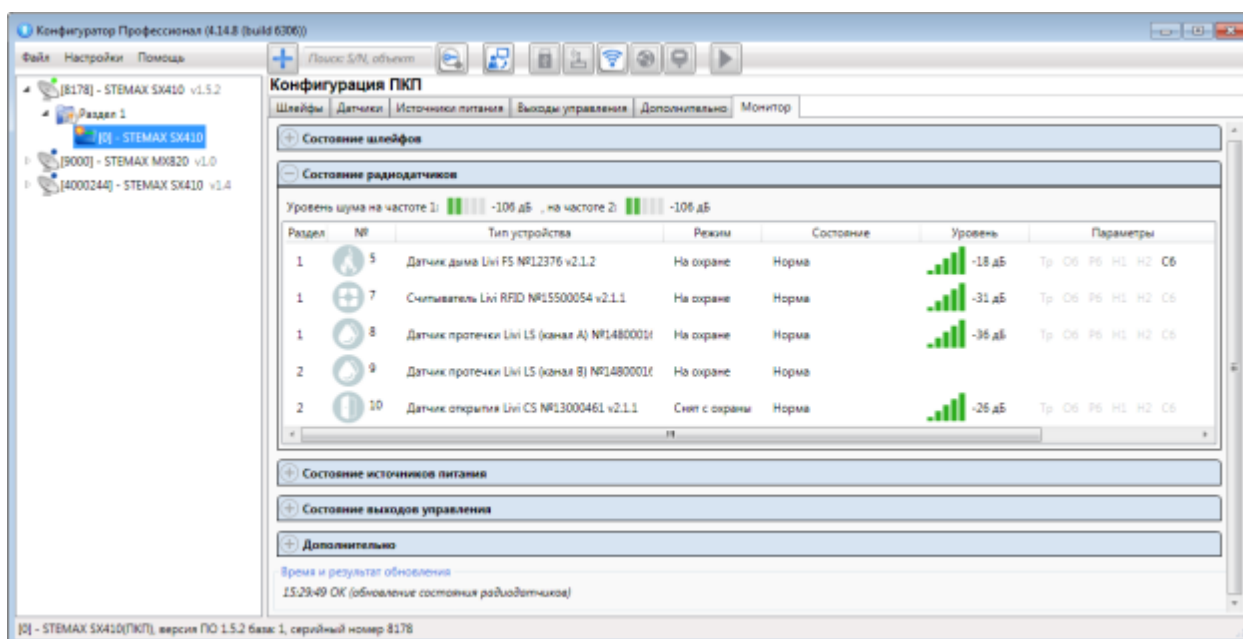
Рис. 5.16. Таблица Состояние радиодатчиков на вкладке Монитор
