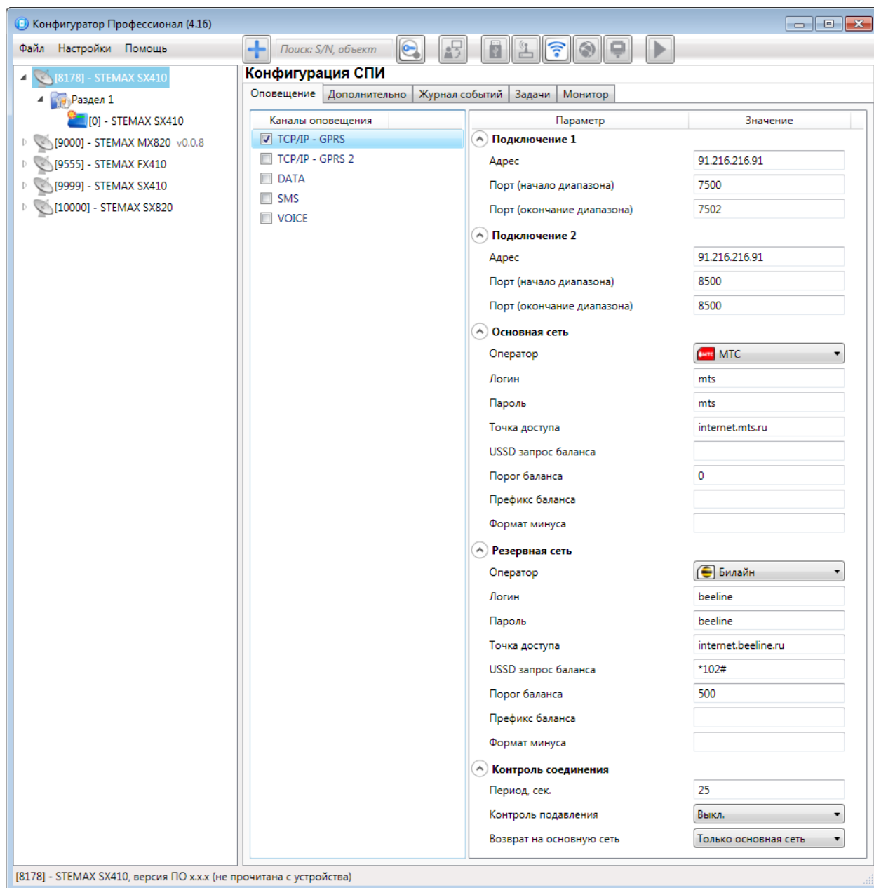
Рис. 5.6. Параметры канала TCP/IP - GPRS
