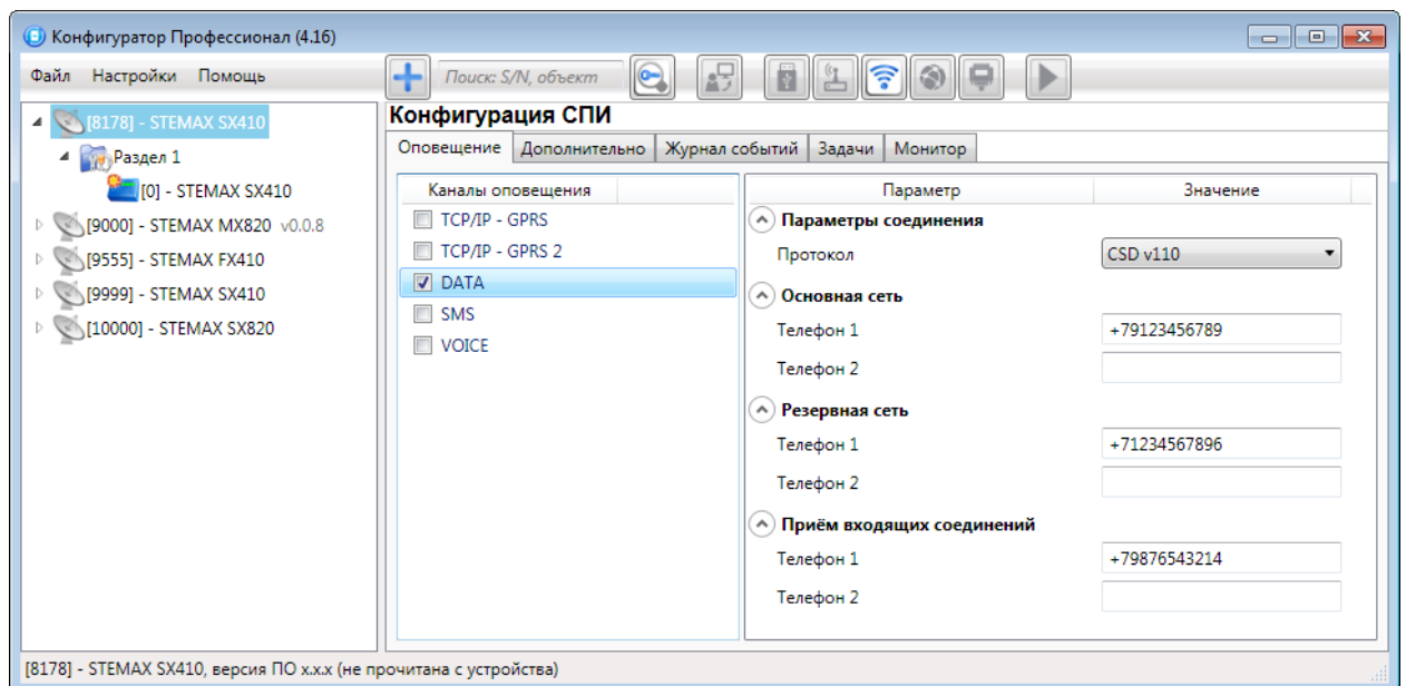
Рис. 5.8. Параметры канала DATA
