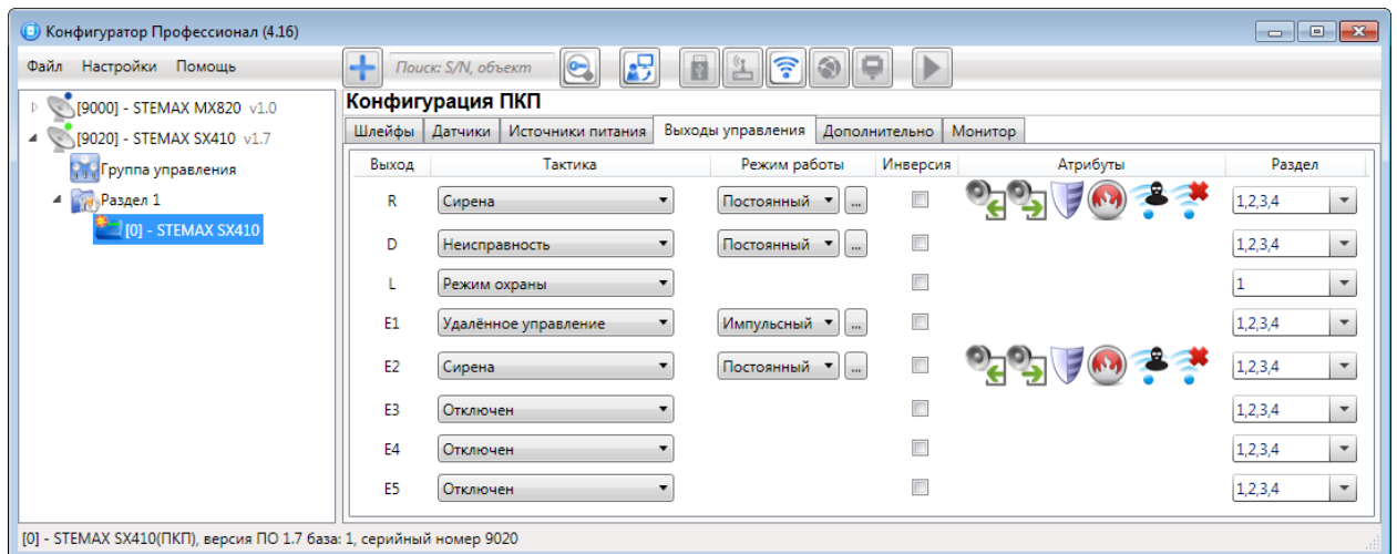
Рис. 5.32. Вкладка Выходы управления
