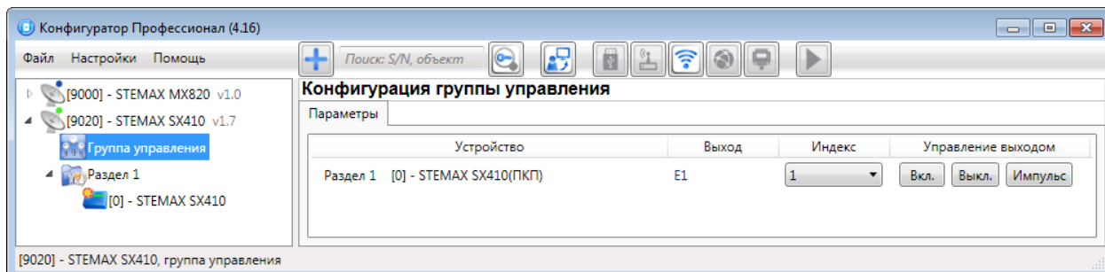
Рис. 5.37. Параметры и элементы дистанционного управления
