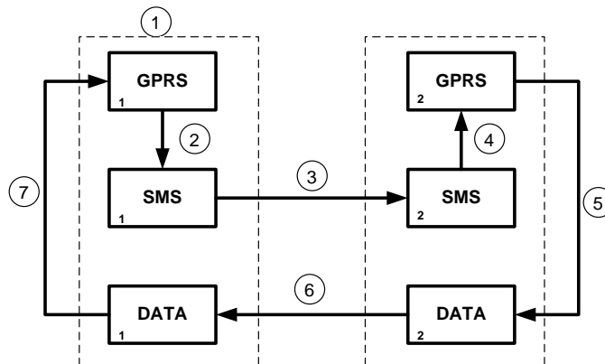
Рис. 3.3. Алгоритм оповещения о тревожных событиях
