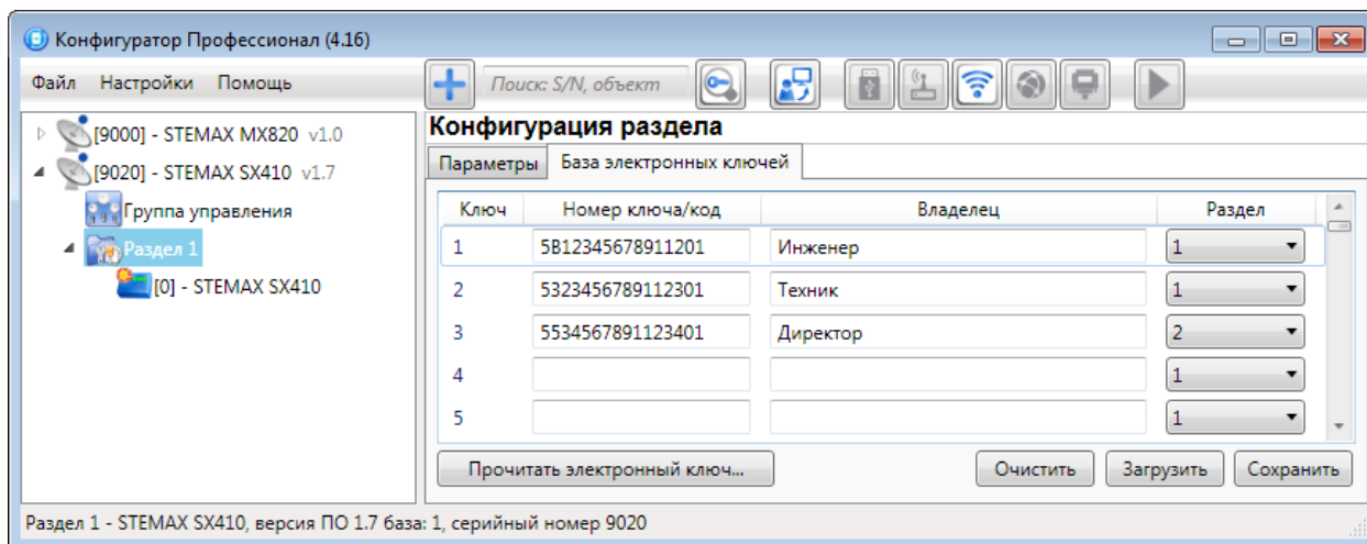
Рис. 5.22. Вкладка База электронных ключей
